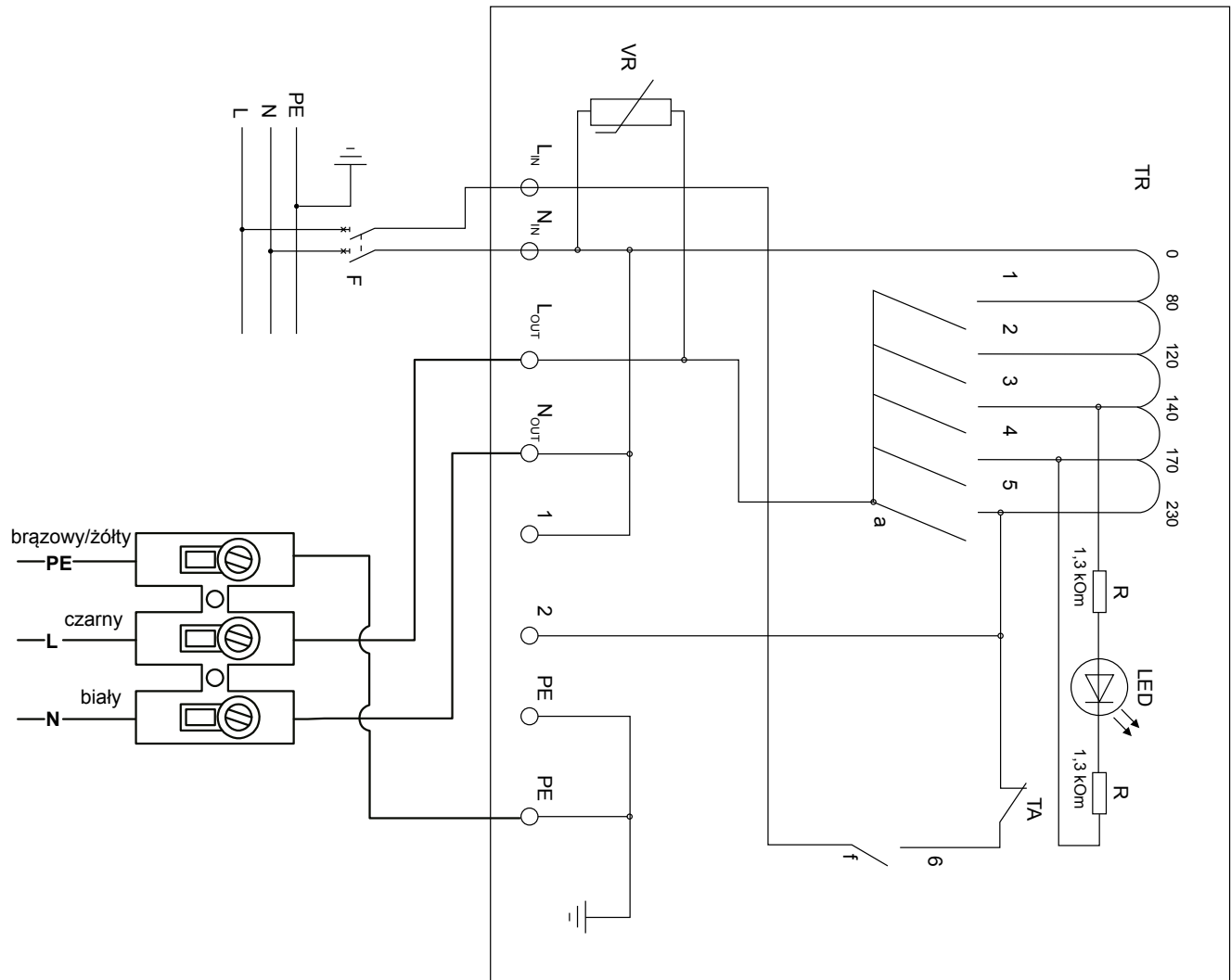
Schemat podłączenia z regulatorem obrotów HRB
