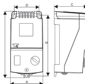
ARW 1,5/1; 3,0; 5,0, 10,0;
