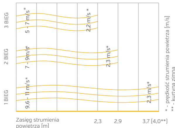
Poziomy zasięg strumienia powietrza (przy montażu pionowym)
